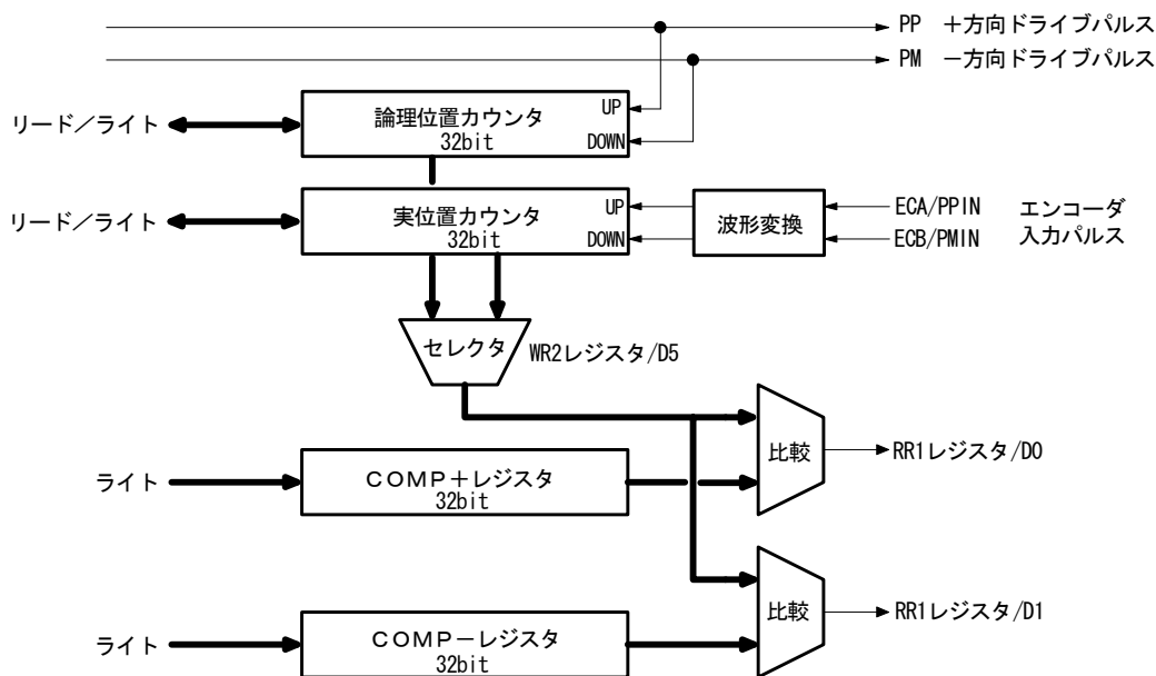
図 2.20 ポジション管理部ブロック構成
