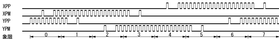
図2.28 円弧補間ドライブパルス出力例
