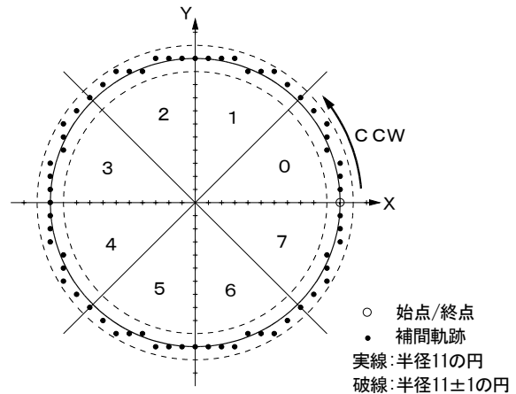
図2.27 円弧補間例
