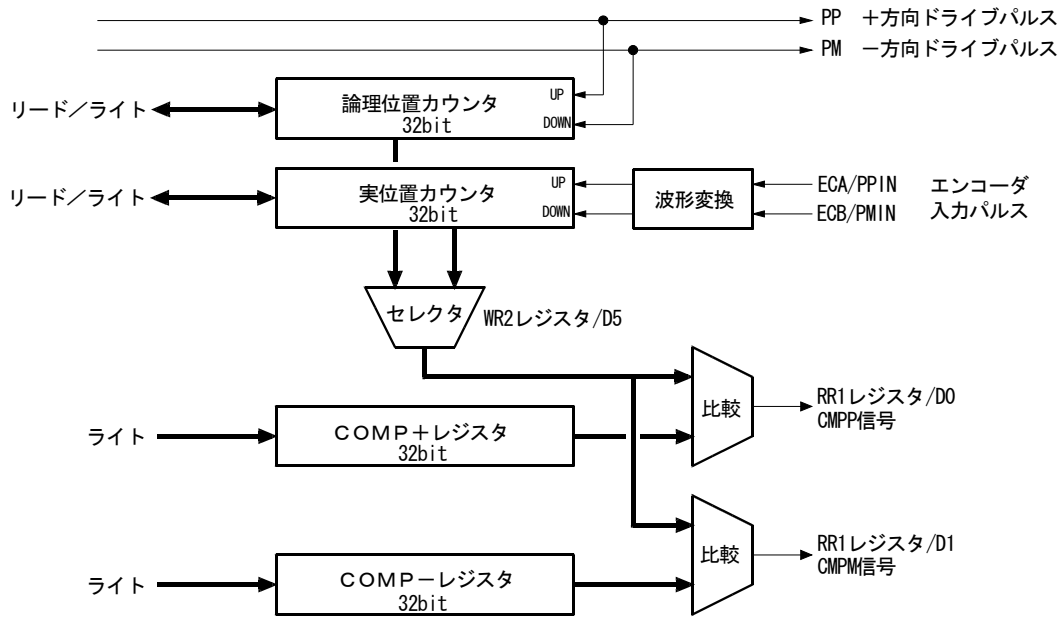
図2.18 ポジション管理部ブロック構成
