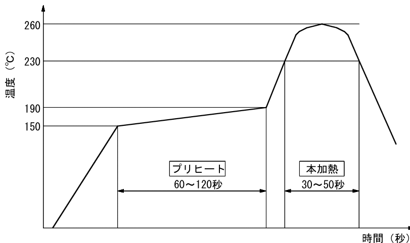
MCX304標準リフロー耐熱温度プロファイル
