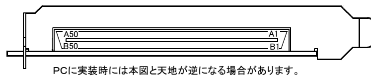
CN2コネクタ ピン配置
