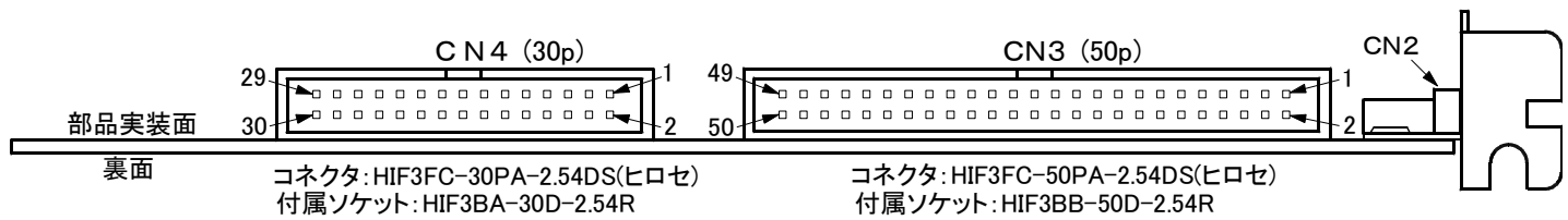
CN3, 4コネクタ ピン配置
