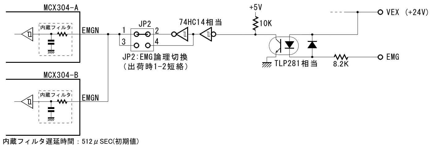
緊急停止入力信号回路
