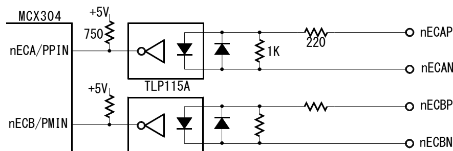
エンコーダA/B相入力信号回路
