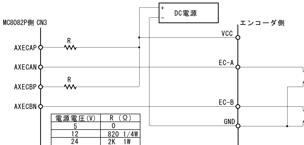
オープンコレクタ出力との接続例
