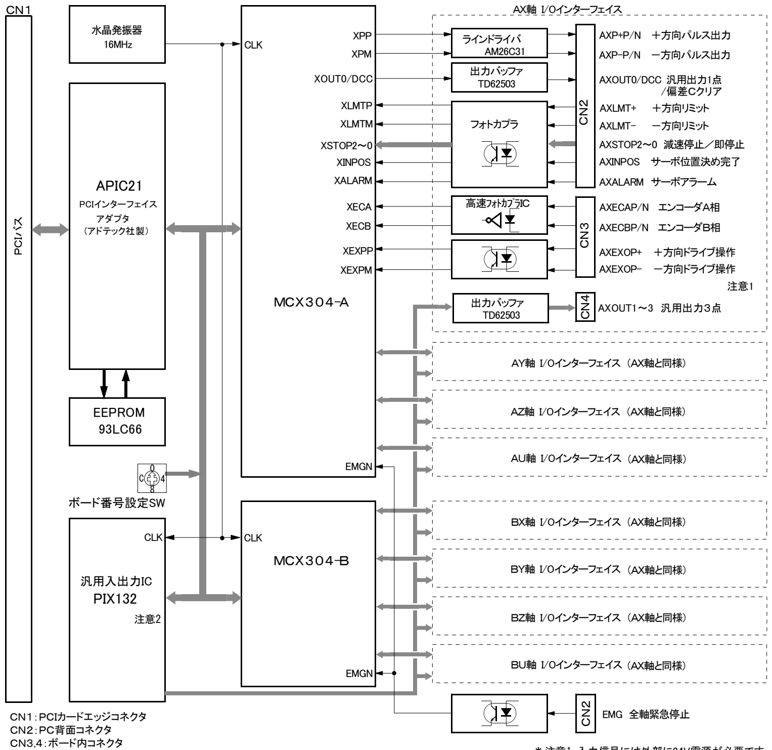
MC8082P 回路ブロック図
