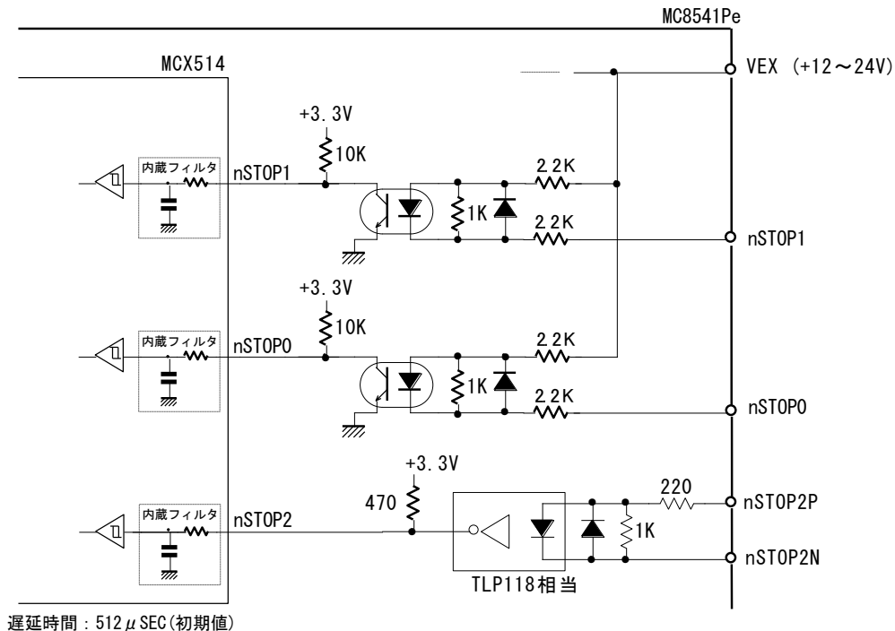
停止入力信号回路
