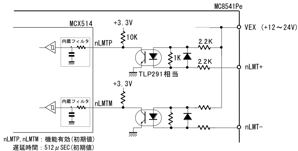
オーバランリミット入力信号回路
