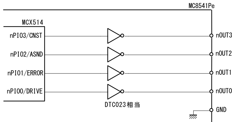
汎用出力信号回路
