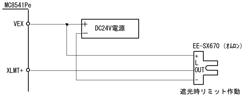
オーバーランリミット入力信号とフォトマイクロセンサとの接続例
