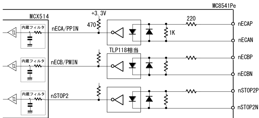
エンコーダ入力信号回路
