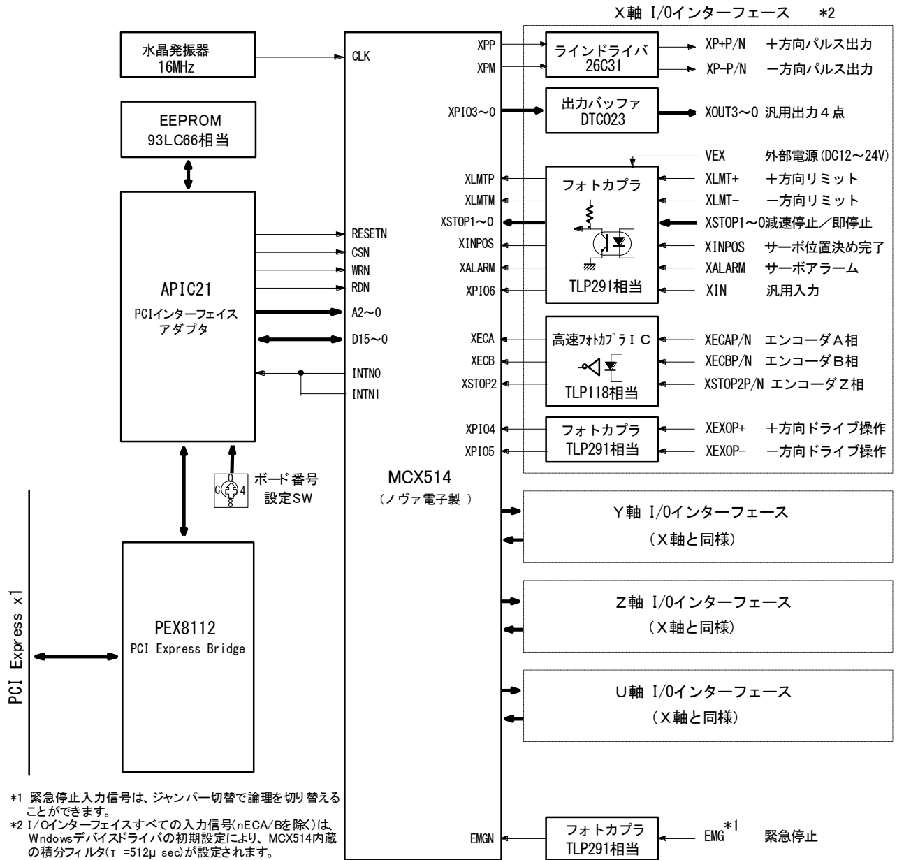
MC8541Pe 回路ブロック図
